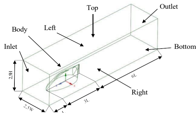
Gambar 4. Pembuatan Fluid Domain
