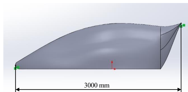
Gambar 1. Panjang (L) Desain Body Kendaraan
