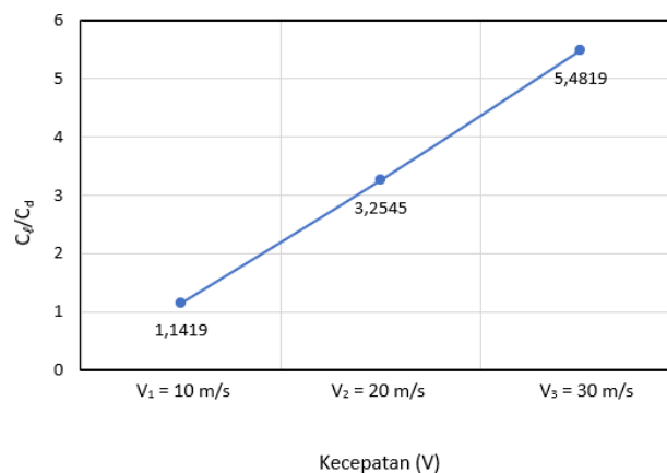
Gambar 11. Grafik rasio C_p/C_d terhadap kecepatan 10 m/s, 20 m/s, dan 30 m/s
