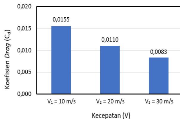
Gambar 6. Perbandingan nilai C_d pada kecepatan 10 m/s, 20 m/s, dan 30 m/s
