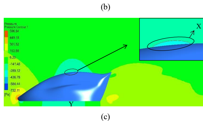
Gambar 10. Pressure contour bagian atas dan bawah pada kecepatan (a) 10 m/s, (b) 20 m/s, dan (c) 30 m/s
