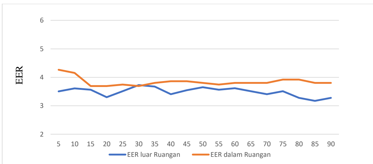
Gambar 7. Grafik Hubungan EER Terhadap Waktu
