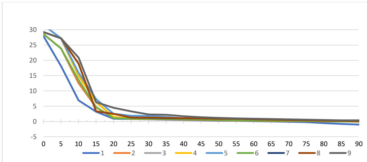
Gambar 5. Grafik Temperatur Produk Terhadap Waktu di Ruang Terbuka
