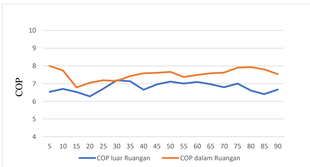
Gambar 6. Grafik Hubungan COP Terhadap Waktu
