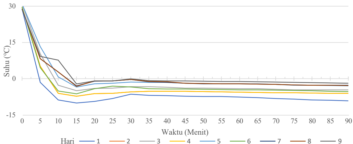
Gambar 3. Grafik Temperature Ruangan di Ruangan Terbuka
