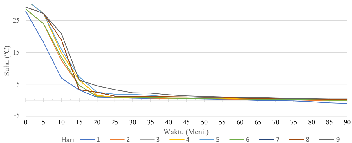
Gambar 5. Grafik Temperatur Produk Terhadap Waktu di Ruangan Terbuka
