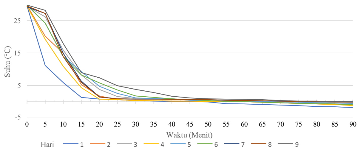
Gambar 4. Grafik Temperature Produk di Ruangan Tertutup
