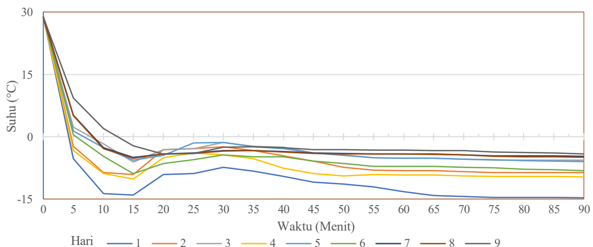
Gambar 2. Grafik Temperature Ruangan di Ruangan Tertutup
