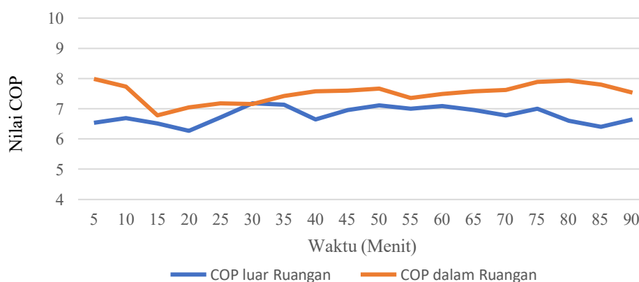
Gambar 6. Grafik Hubungan COP Terhadap Waktu
