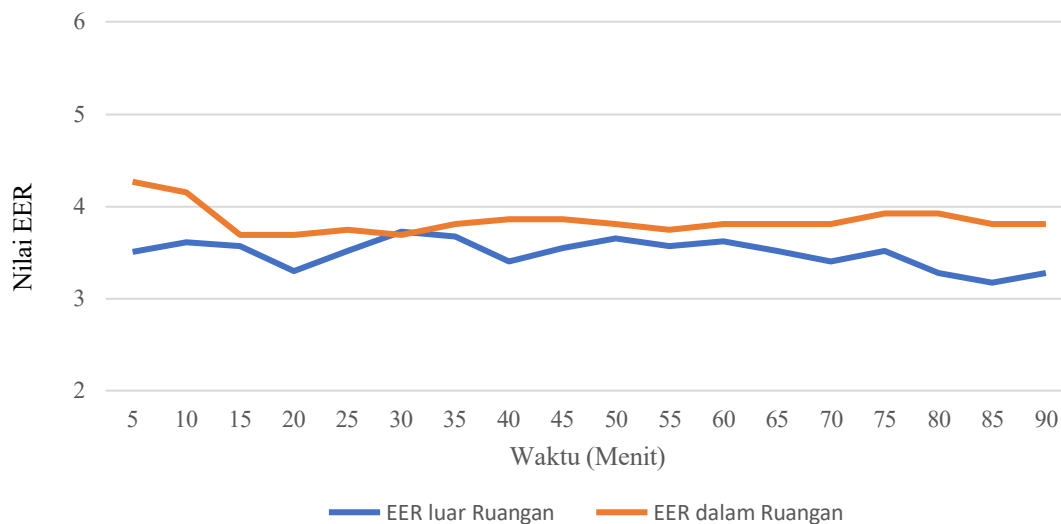
Gambar 7. Grafik Hubungan EER Terhadap Waktu
