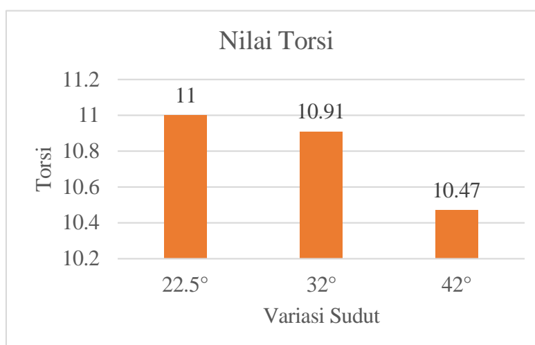
Gambar 6. Perbandingan nilai torsi pada variasi 22,5°, 32°, 42°
